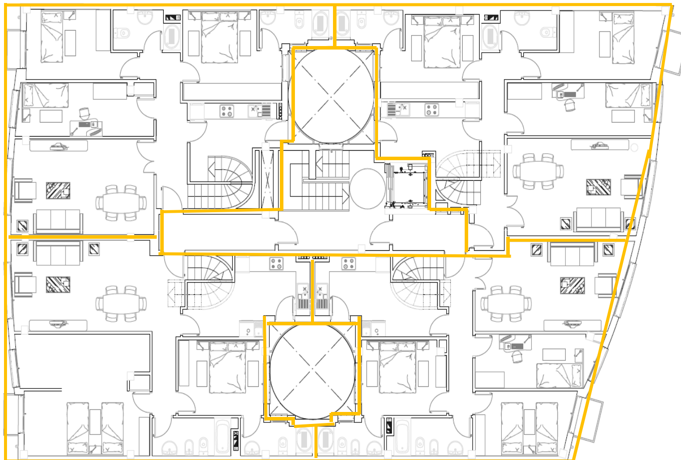
Planta tercera
