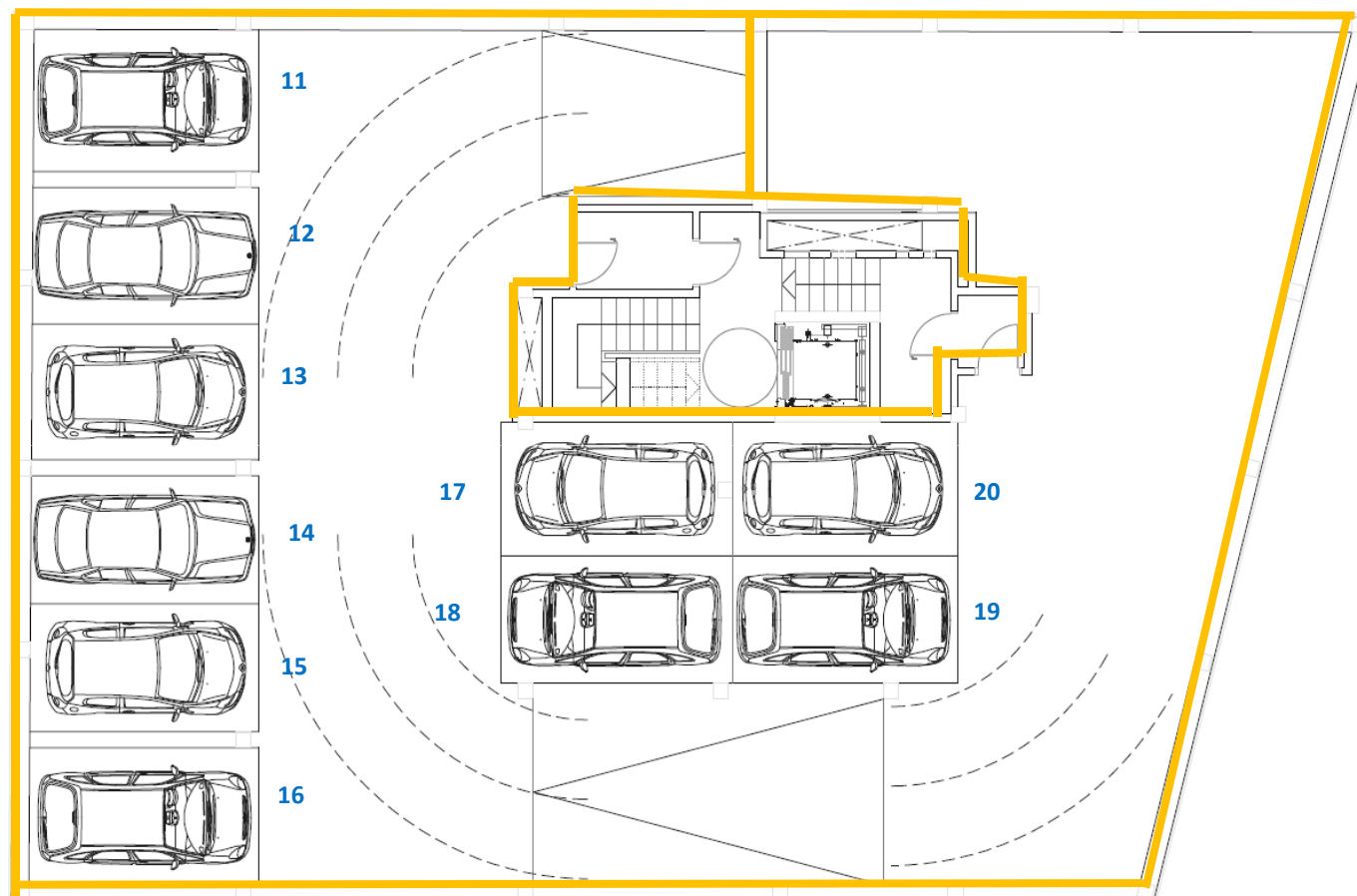
Planta sótano 2
