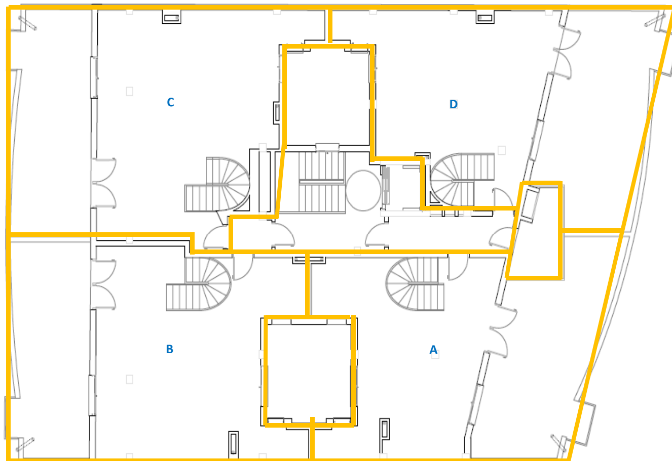
Planta trasteros
